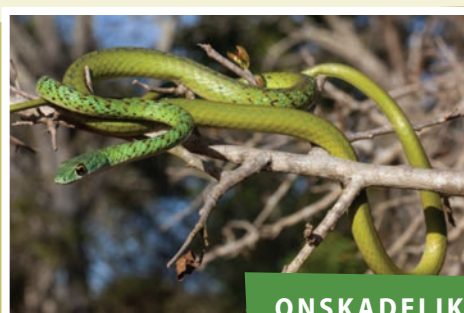
Gespikkelde bosslang ( Philothamnus semivariegatus )
