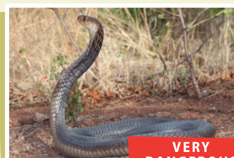
Anchieta's Cobra ( Naja anchietae )
